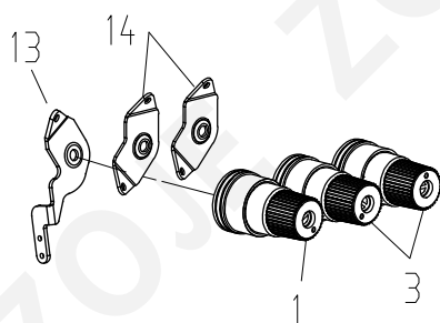
三线调线机构
