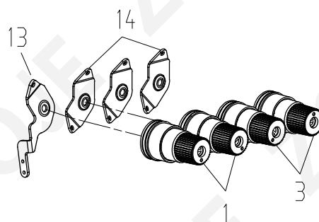
四、五线调线机构
