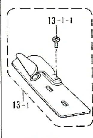
<1/8, 5/32用>
