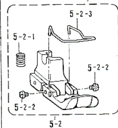
<1/8, 5/32用>
