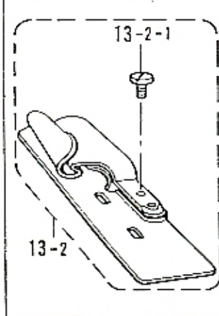
<3/16, 1/4MH用>
