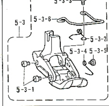
<1/4M用>
