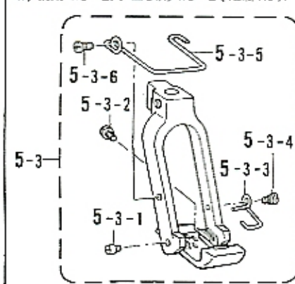
<厚物用>
