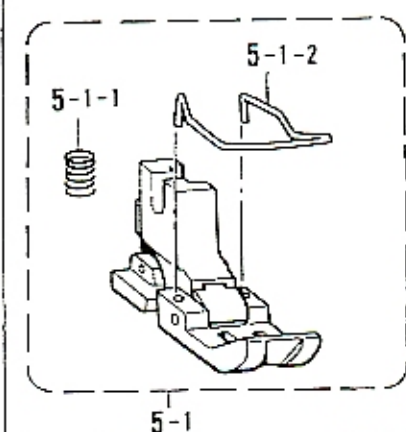
<固定針受用>
