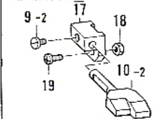
<移動針受用>
