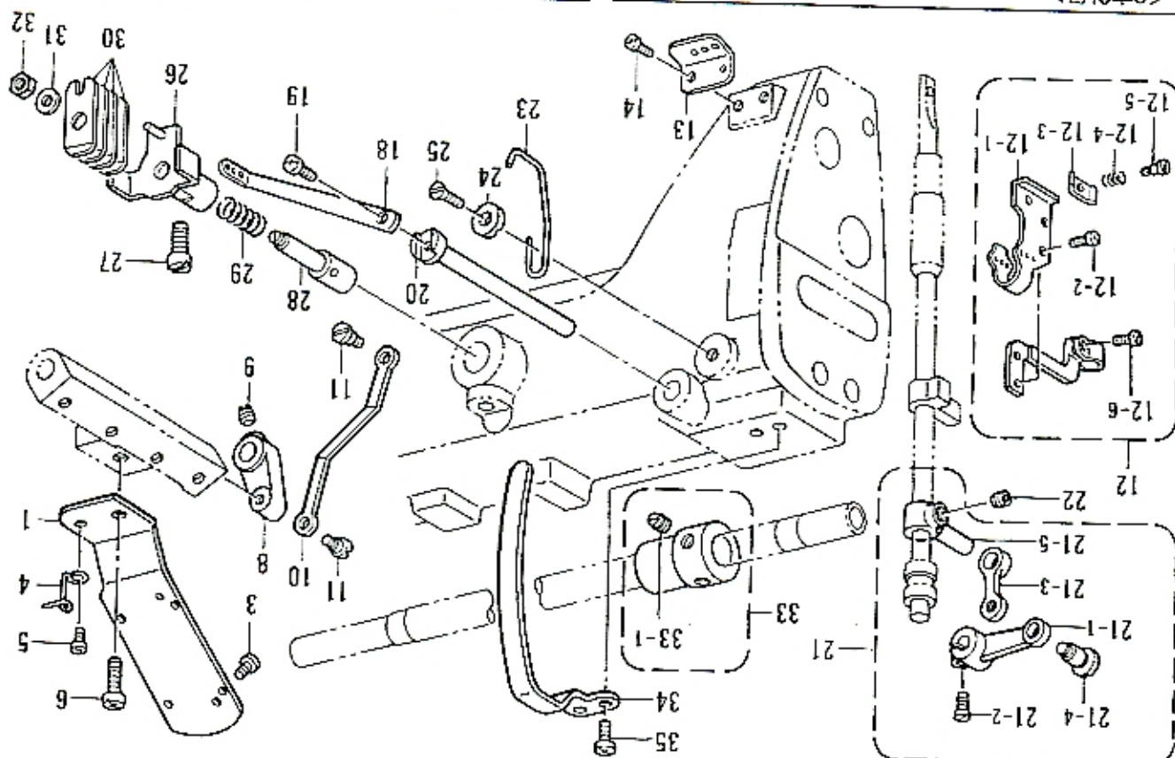
上引線装置(928)/Upper threading mechanism(928)
